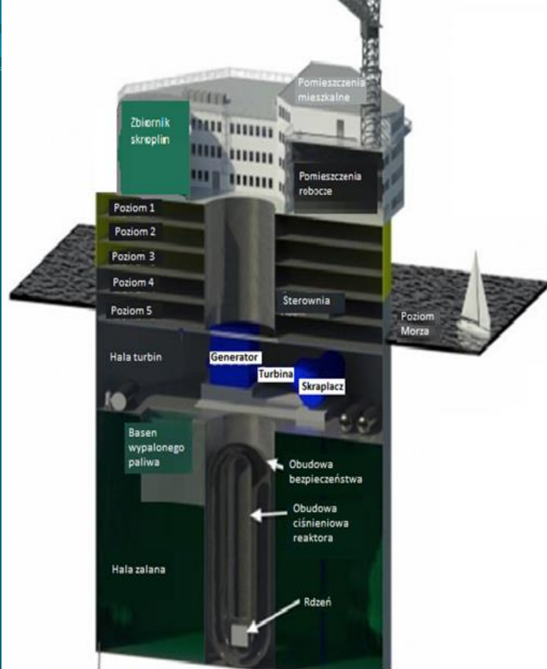
Wizja elektrowni pływającej na platformie (MIT news Office)
